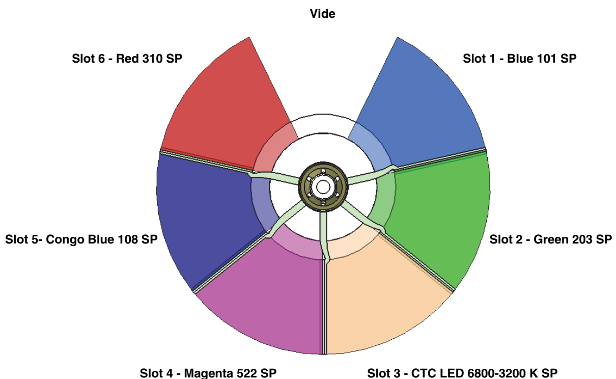
Figure 1: Roue de couleur du MAC Quantum Profile
