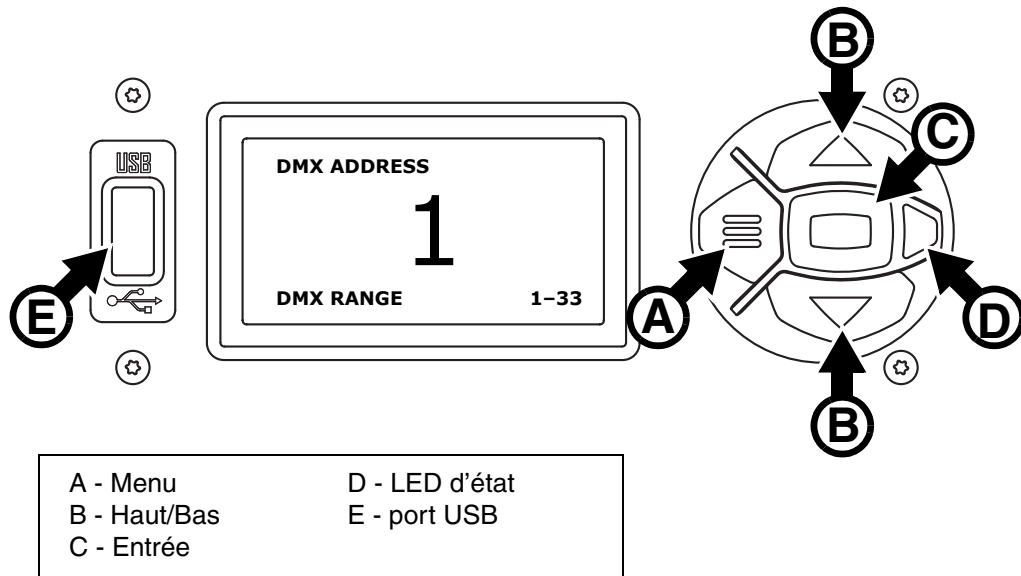
Figure 5: Panneau de contrôle et afficheur
