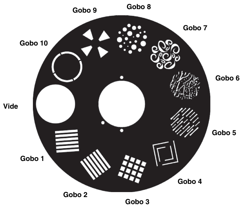
Figure 2: Roue de gobos fixes du MAC Quantum Profile
