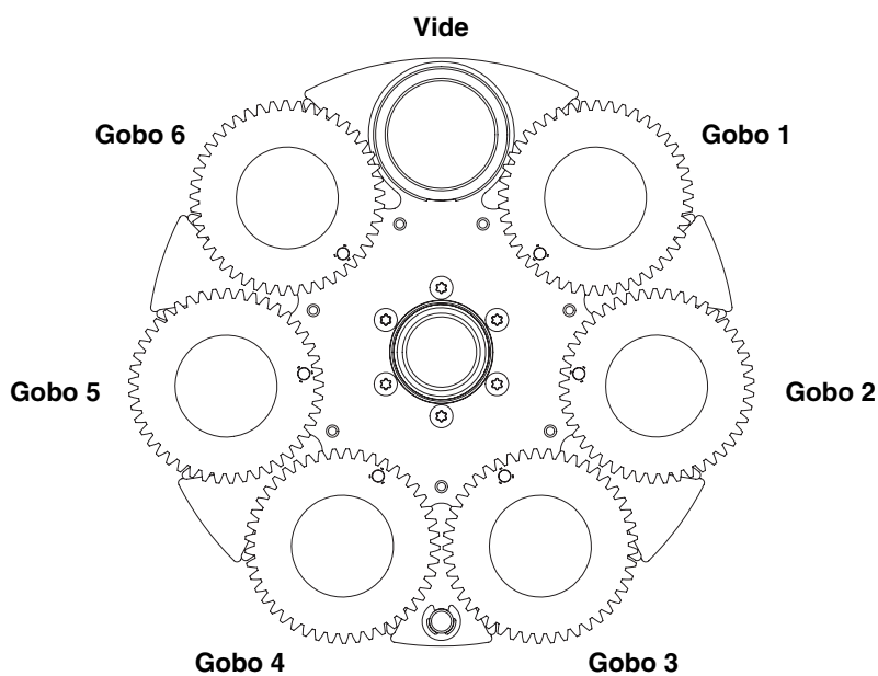
Figure 3: Roue de gobos tournants du MAC Quantum Profile
